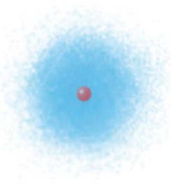
Mô hình (2) của nguyên tử hydrogen
